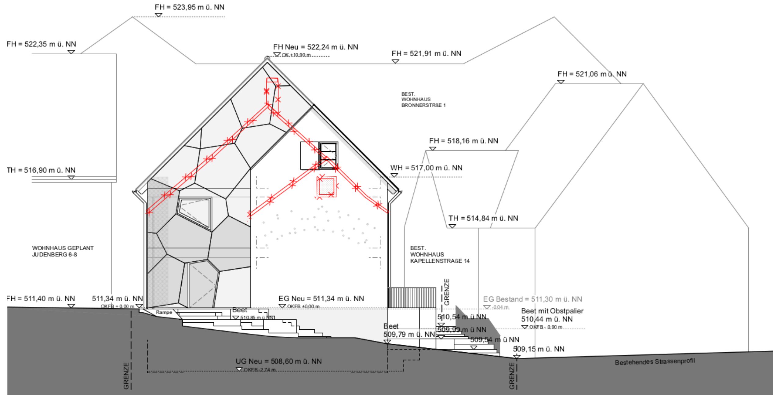
Ansicht Norden
