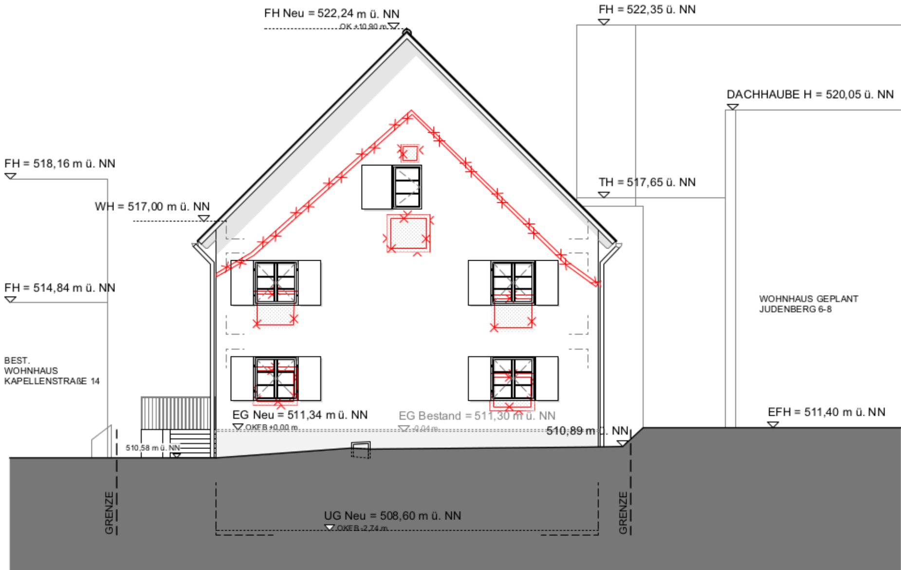
Ansicht Süden
