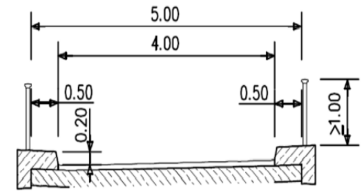
Bild 2.1.1: Querschnittsbreite von Überführungen ländlicher Wege
